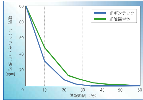
アセトアルデヒド分解能力比較
